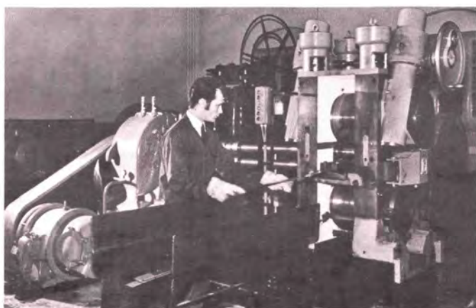
Walsmachine voor het op dikte pletten van metaalstro- ken
