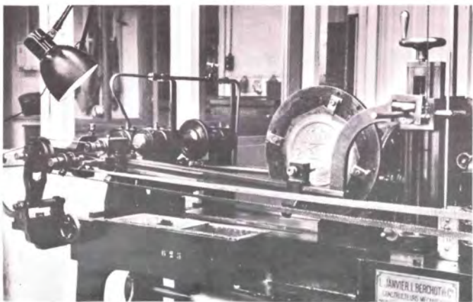
Verkleinbank voor het verkleinend overbrengen van een bronzen model op schaal
